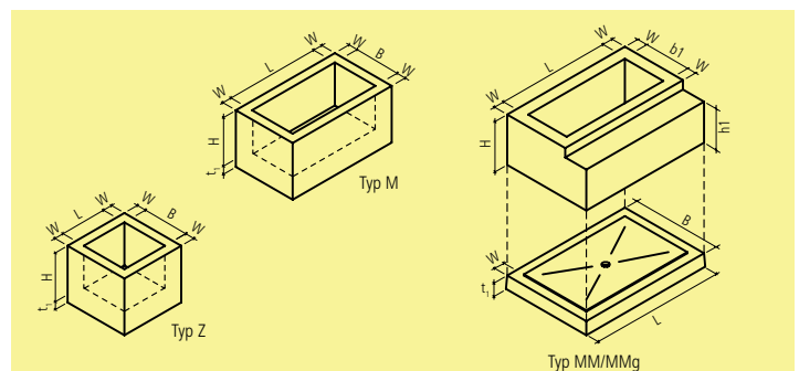
Kabelschächte quadratisch/rechteckig
