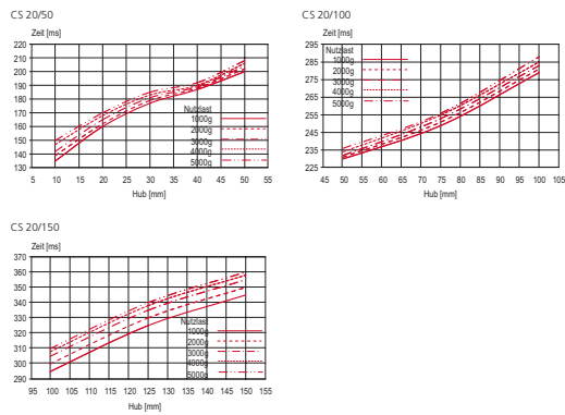
Verfahrzeit-Diagramme
